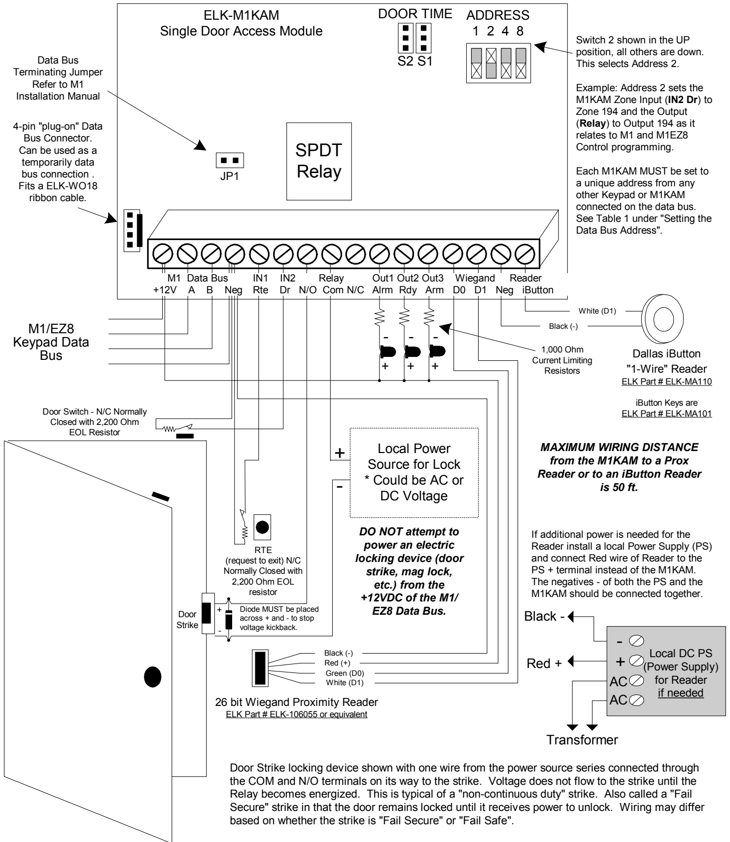
Hookup Diagram for ELK-M1KAM Single Door Access Module
